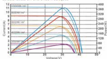
características em diferentes irradiações
